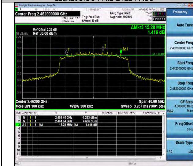
11ax20ISO-Ant1-2462-PASS
