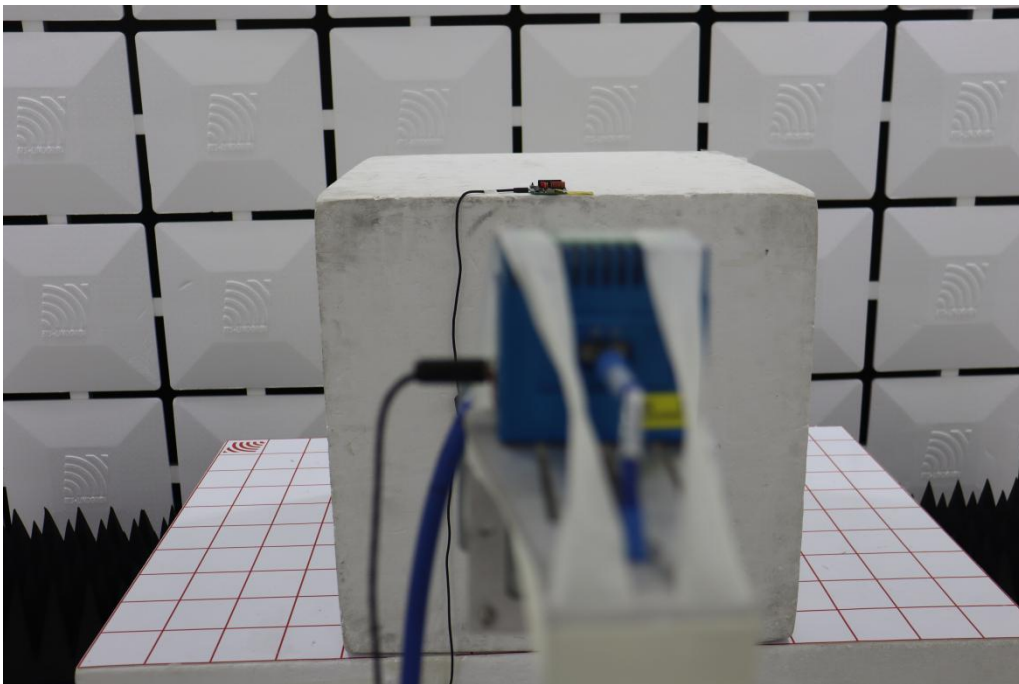
Above 18GHz
