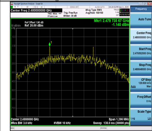
BLE 500K-Ant1-2480-PASS
