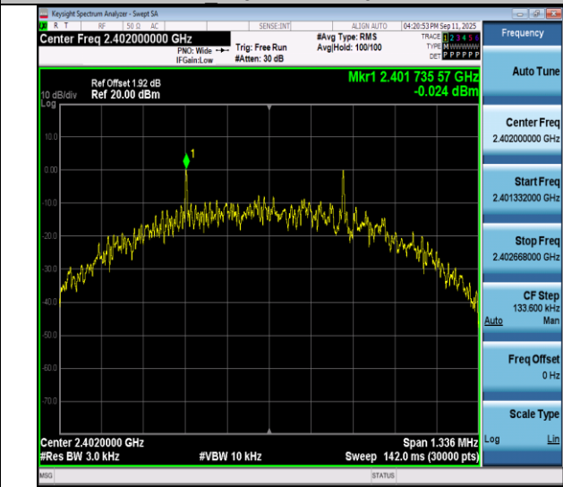
BLE 500K-Ant1-2402-PASS
