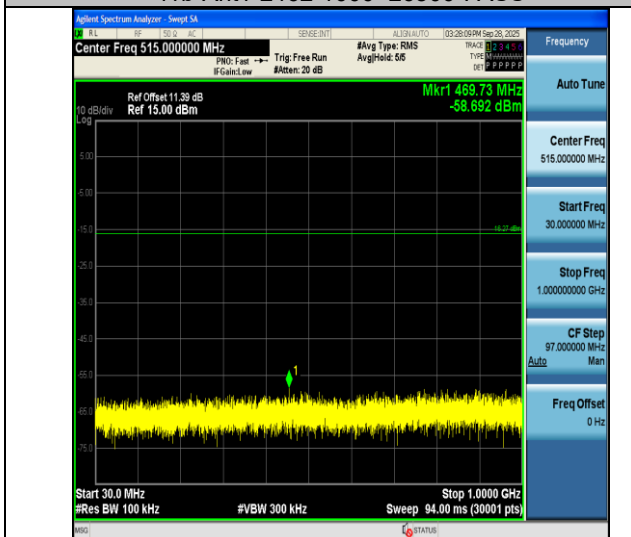
11g-Ant1-2412-30~1000-PASS
