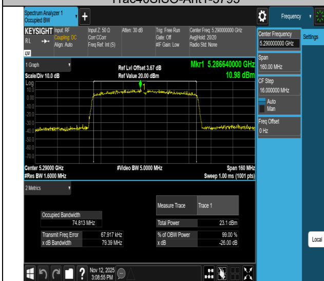
11ac80SISO-Ant1-5290
