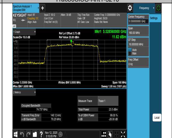
11ac80SISO-Ant1-5530
