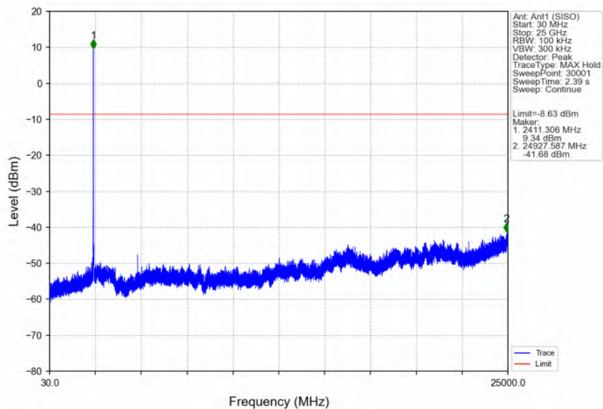
802.11b_LCH_2412MHz_Ant1 (SISO)_NTNV
