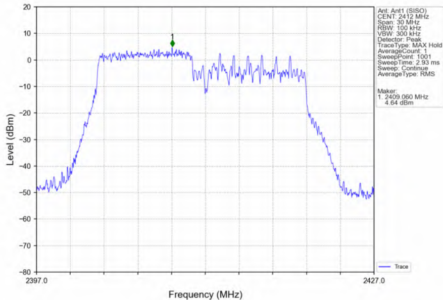
802.11ax(HEW20)_LCH_2412MHz_RU106_Left_Ant1 (SISO)_NTNV
