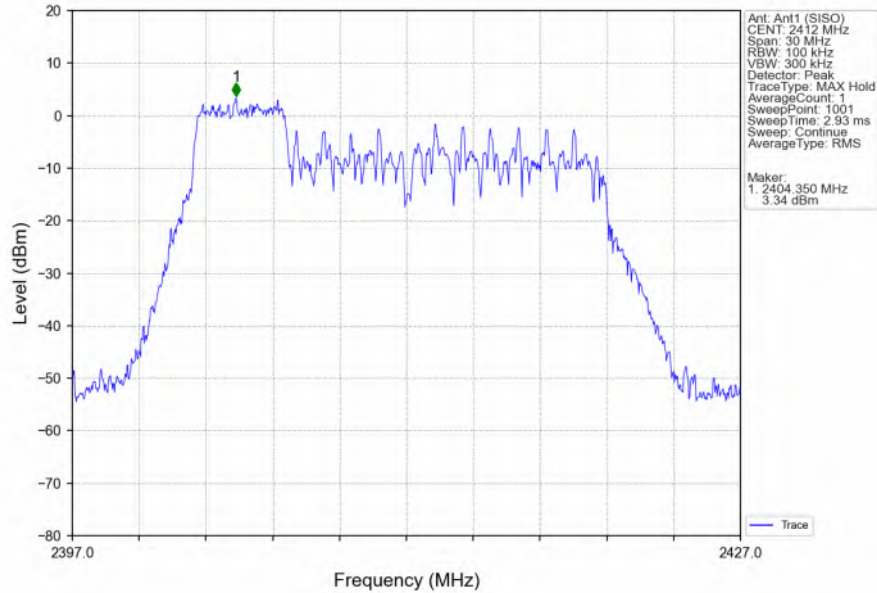
802.11ax(HEW20)_LCH_2412MHz_RU106_Left_Ant1 (SISO)_NTNV
