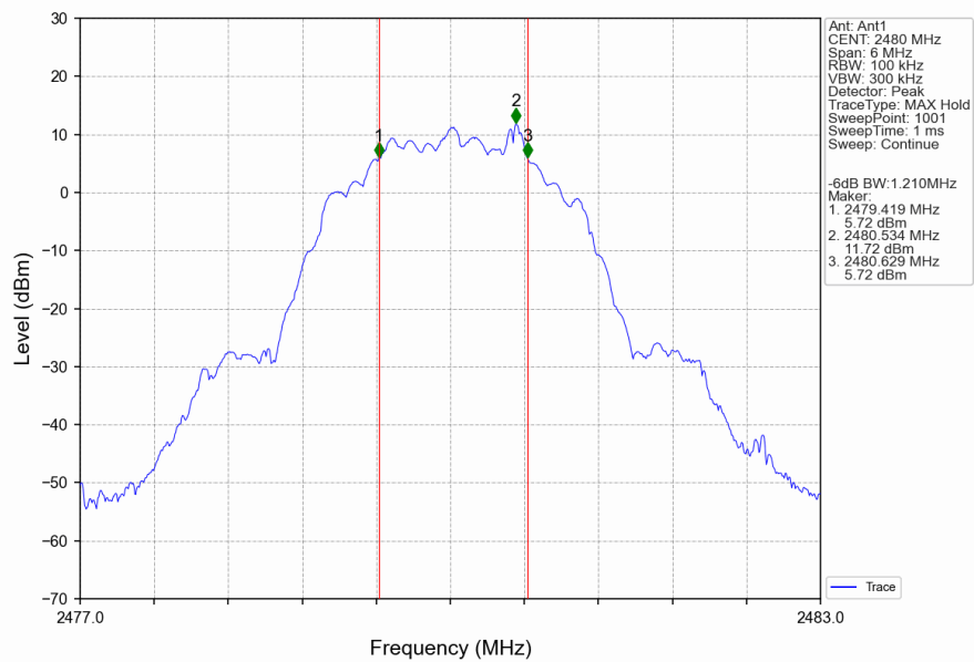
2M_HCH_2480MHz_Ant1_NTNV
