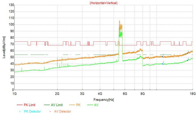
11N_40M_5670
