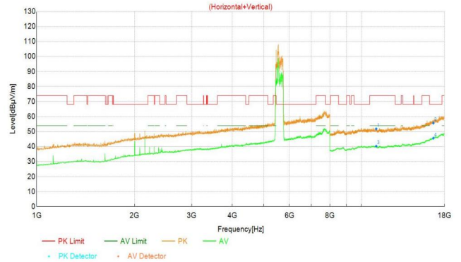
11N_40M_5710
