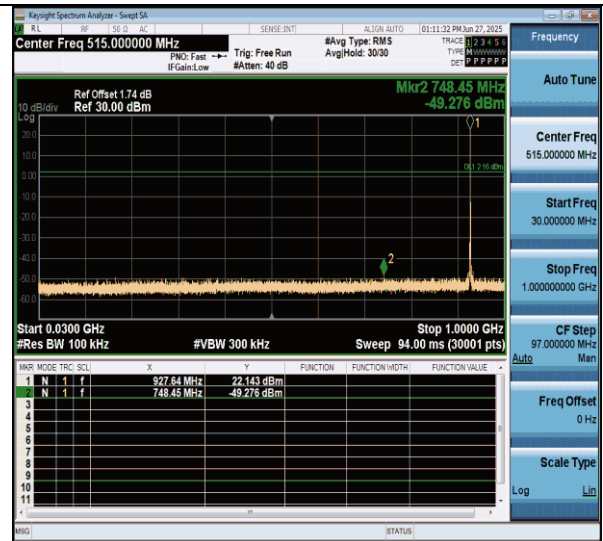
LORA_DSS-Ant1-927.6-30~1000-PASS
