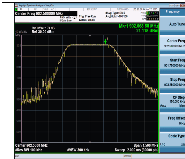
LORA_DTS-Ant1-902.5-PASS
