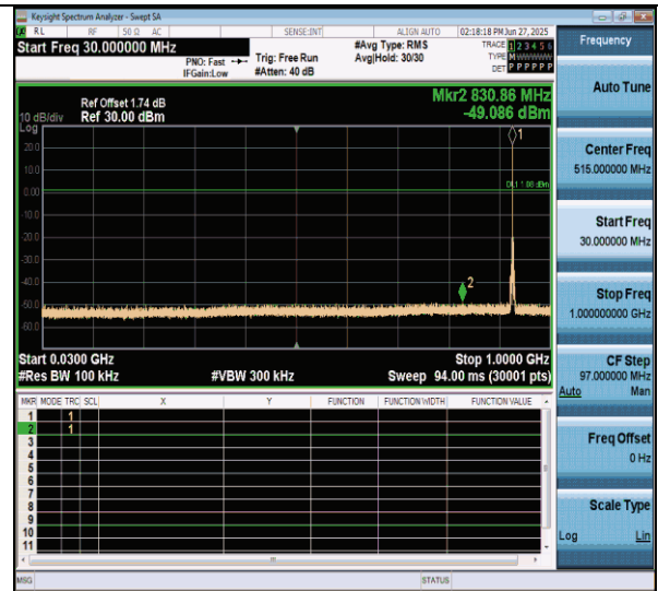
LORA_DTS-Ant1-926.5-30~1000-PASS
