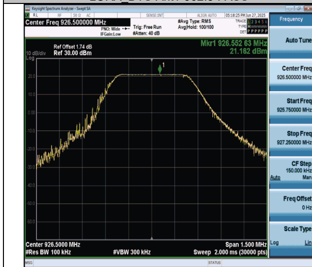
LORA_DTS-Ant1-926.5-PASS
