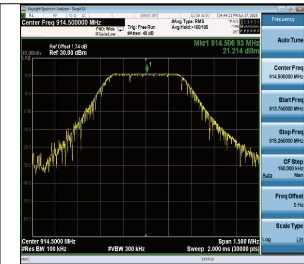
LORA_DTS-Ant1-914.5-PASS
