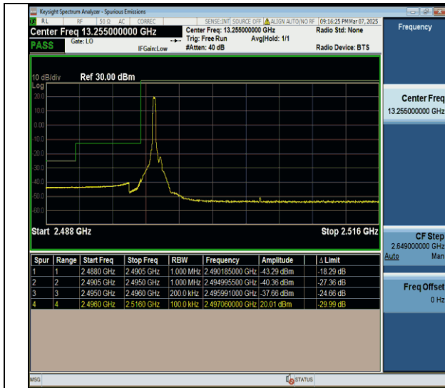
Band41-20MHz-QSPK-39750-1RB#0-PASS
