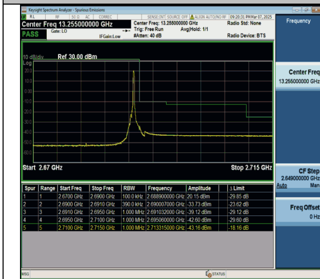
Band41-20MHz-QSPK-41490-1RB#99-PASS
