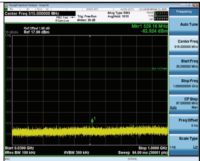
11n20SISO-Ant0-2462-30-1000-PASS
