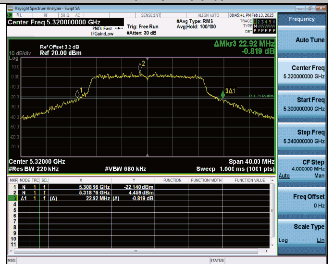
11ac20SISO-Ant0-5320
