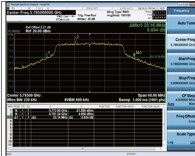
11n20SISO-Ant0-5785
