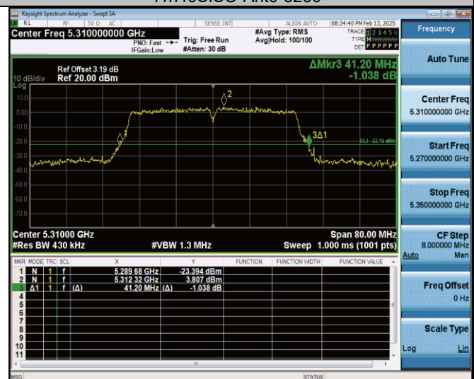
11n40SISO-Ant0-5310
