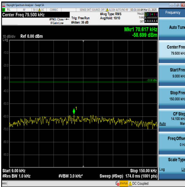
Band71-20MHz-QPSK-133372-1RB#0-0.009~0.15-PASS
