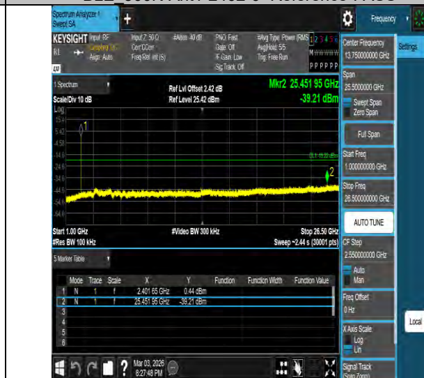
BLE 500K-Ant1-2402-1000~26500-PASS
