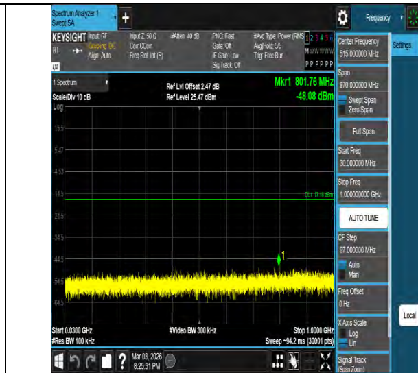
BLE 125K-Ant1-2480-30~1000-PASS
