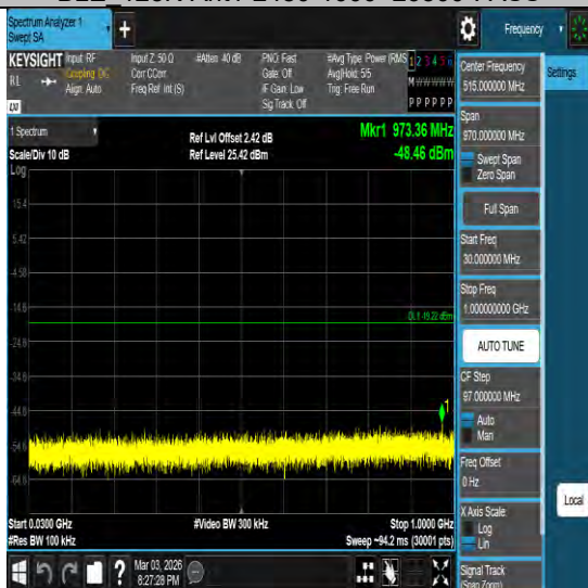
BLE 500K-Ant1-2402-30~1000-PASS
