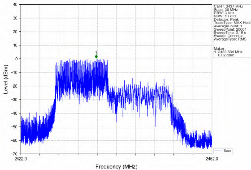
802.11ax(HEW20) MCH_2437MHz_RU106_Ant1 (SISO) NTNv
