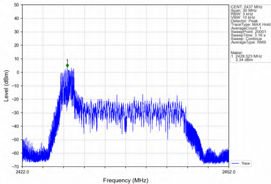
802.11ax(HEW20) MCH_2437MHz_RU26_Ant1 (SISO) NTN
