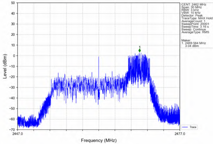
802.11ax(HEW20) HCH_2462MHz_RU106_Ant1 (SISO) NTNv
