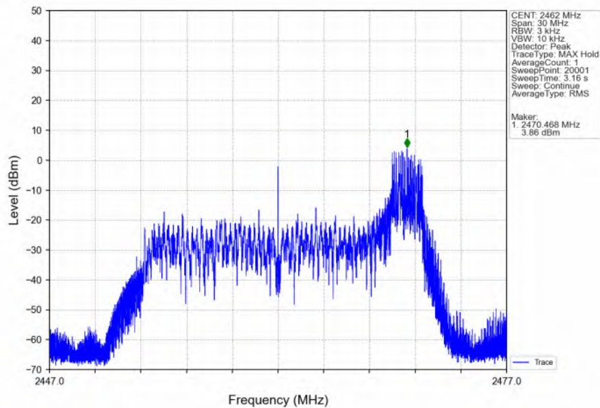
802.11ax(HEW20) HCH 2462MHz RU26 Ant1 (SISO) NTN
