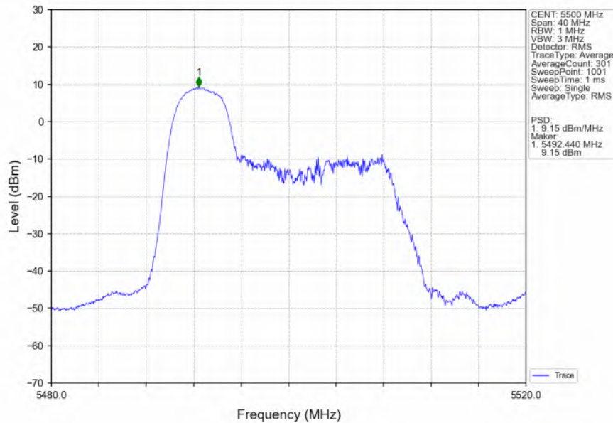
802.11ax(HEW20)_LCH_5500MHz_RU106_Ant1_NTNV
