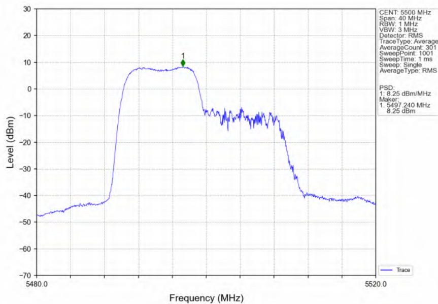
802.11ax(HEW20)_LCH_5500MHz_RU106_Ant1_NTNV
