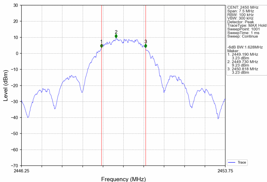
802.15.4 (Thread/Zigbee) MCH 2450MHz Ant1 NTN
