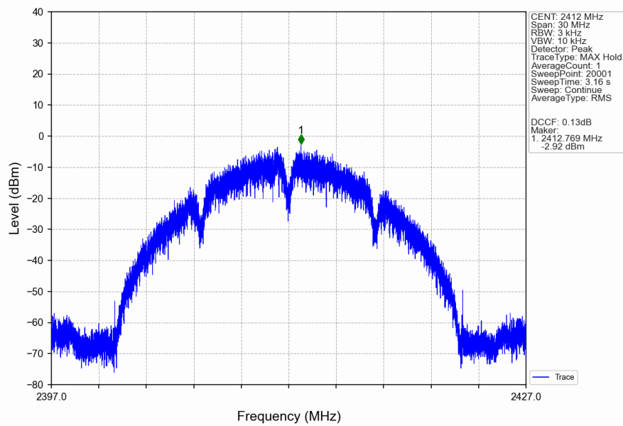
802.11b_LCH_2412MHz_Ant1 (MIMO)_NTNV
