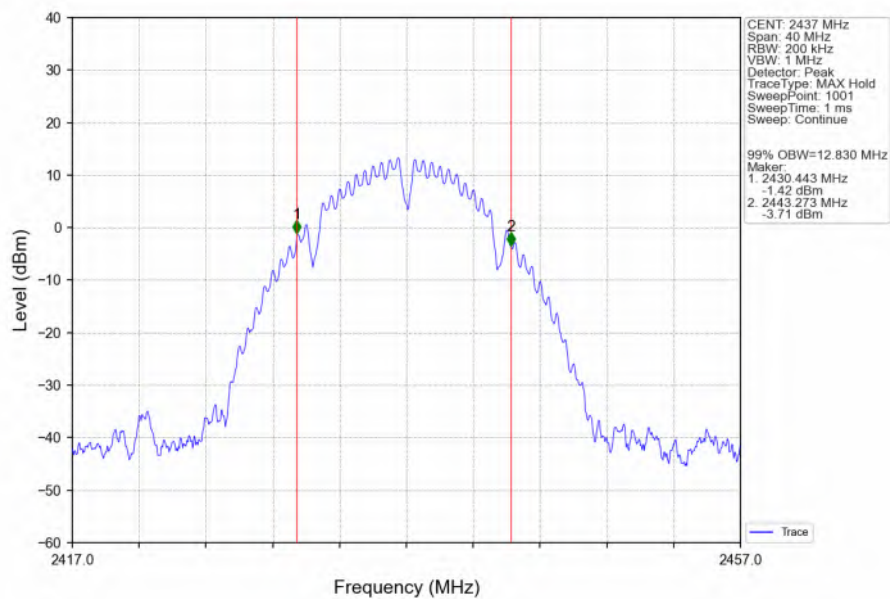
802.11b_MCH_2437MHz_Ant0 (MIMO)_NTNV
