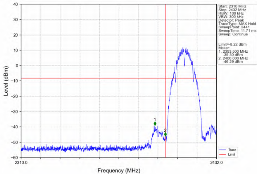
802.11b_LCH_2412MHz_Ant0 (MIMO)_NTNV
