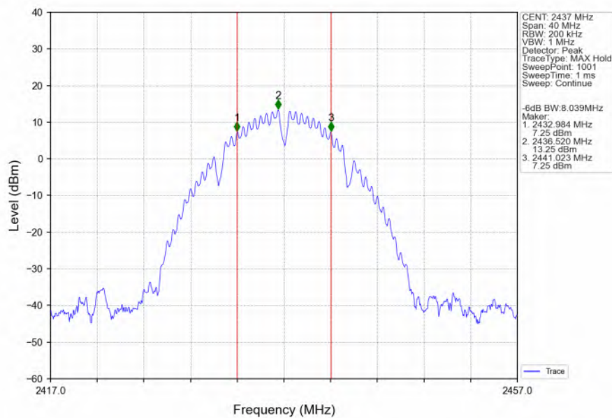
802.11b_MCH_2437MHz_Ant0 (MIMO)_NTNV
