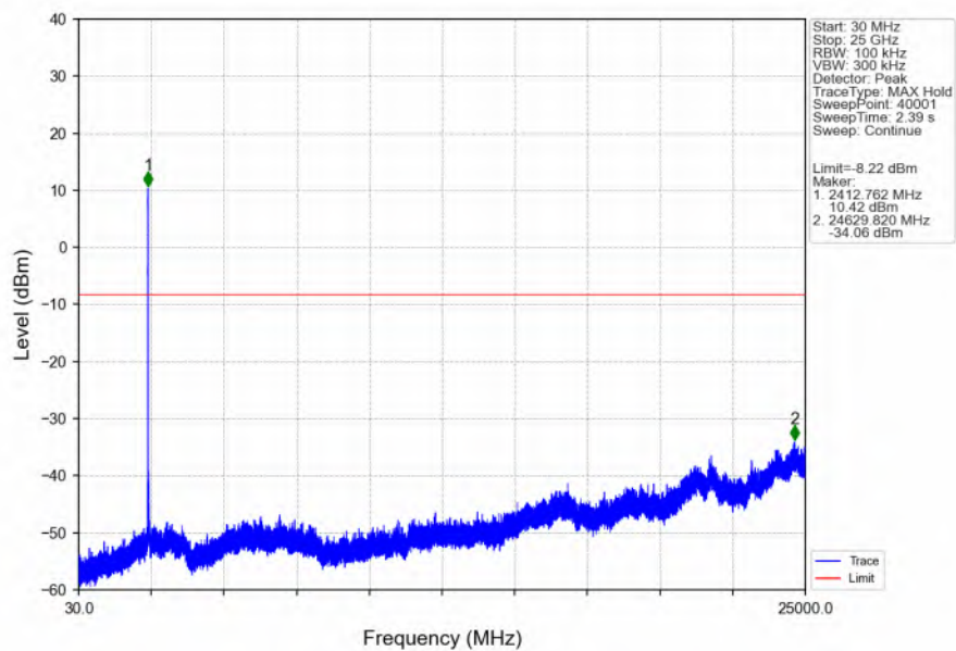
802.11b_LCH_2412MHz_Ant0 (MIMO)_NTNV
