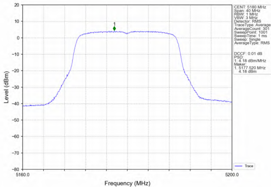
802.11be(EHT20)_LCH_5180MHz_SU_/_Ant1_NTNV
