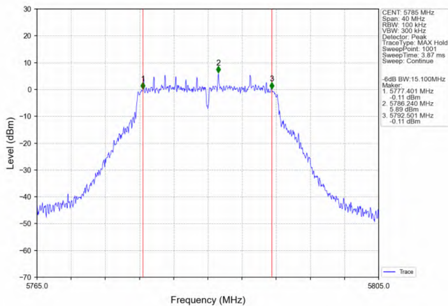
802.11a_MCH_5785MHz_Ant0_NTNV
