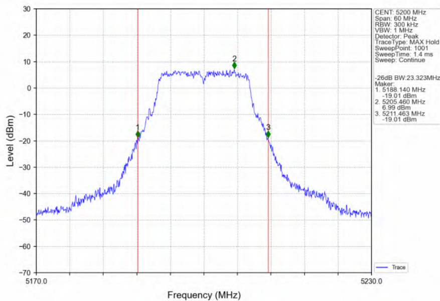
802.11a_MCH_5200MHz_Ant0_NTNV
