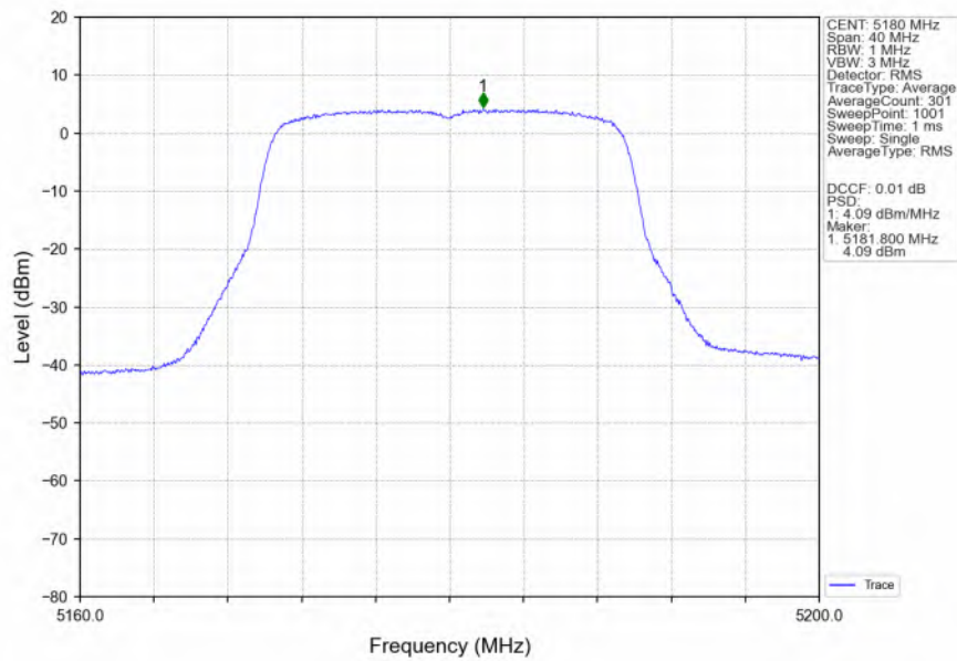
802.11be(EHT20)_LCH_5180MHz_SU_/_Ant1_NTNV
