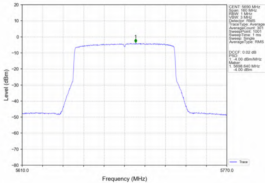
802.11be(EHT80)_HCH_5690MHz_SU_/_Ant1_NTNV
