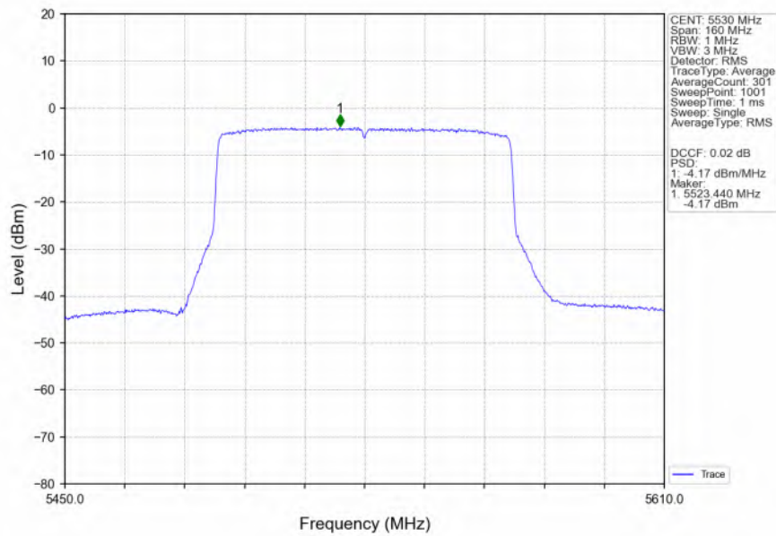
802.11be(EHT80)_LCH_5530MHz_SU_ / _Ant1_NTNV
