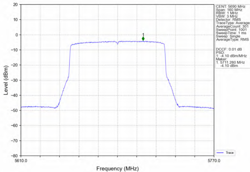
802.11be(EHT80)_HCH_5690MHz_SU_/_Ant1_NTNV
