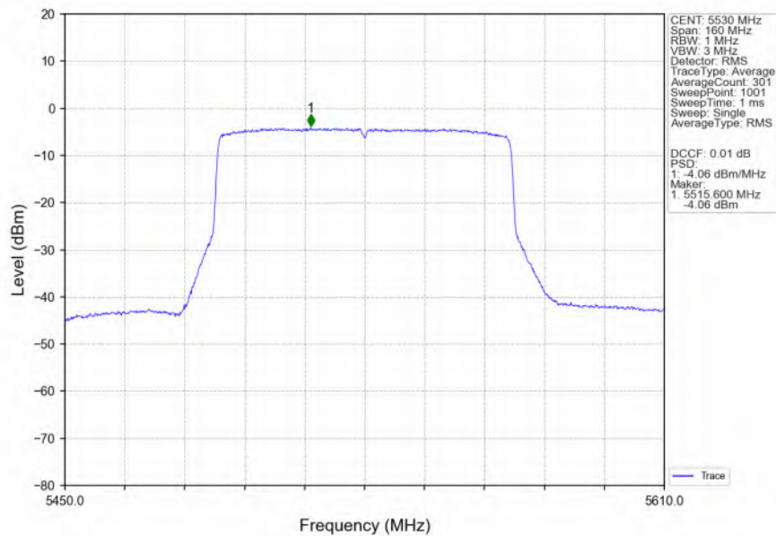
802.11be(EHT80)_LCH_5530MHz_SU_ / _Ant1_NTNV
