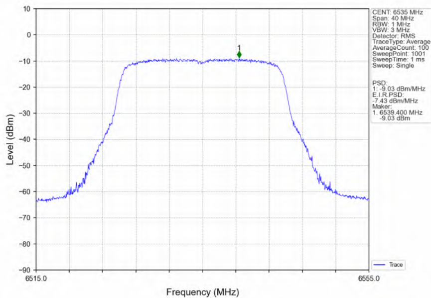
802.11be(EHT20)_LCH_6535MHz_SU_/_Ant1_NTNV
