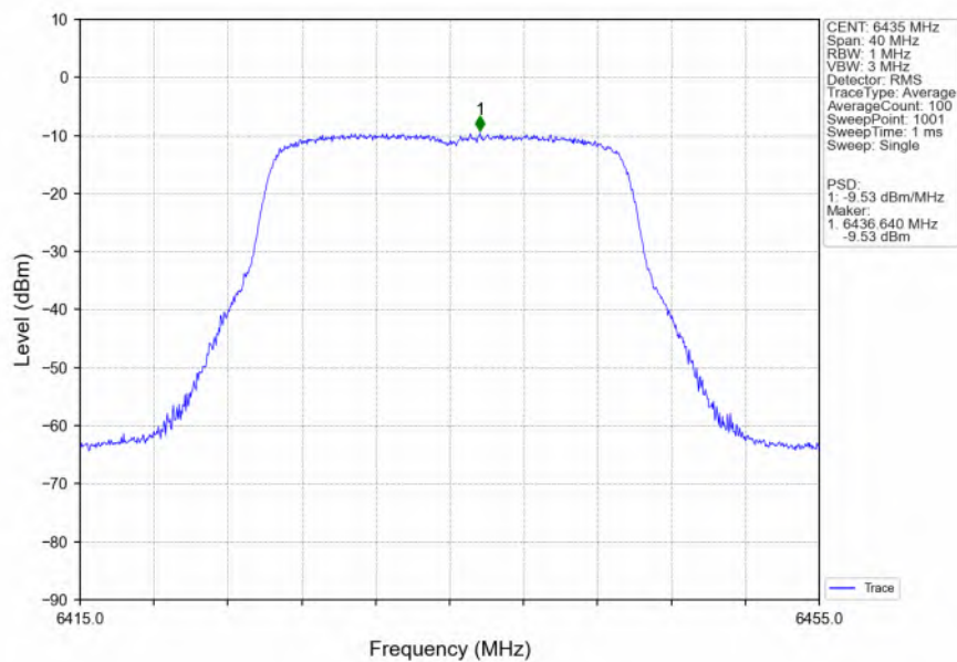
802.11be(EHT20)_LCH_6435MHz_SU_/_Ant1_NTNV
