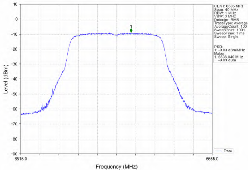
802.11be(EHT20)_LCH_6535MHz_SU_/_Ant1_NTNV
