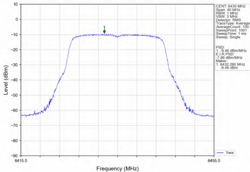
802.11be(EHT20)_LCH_6435MHz_SU_/_Ant1_NTNV
