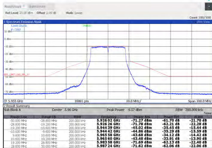
11a-CDD_Ant1_5955
