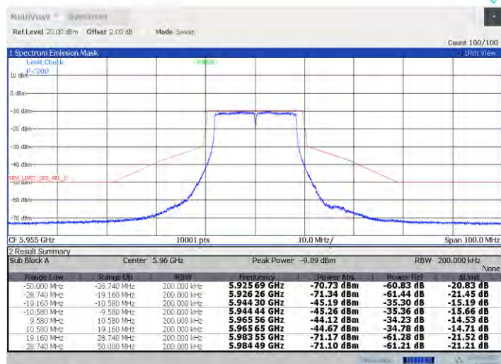
11a-CDD_Ant1_5955
