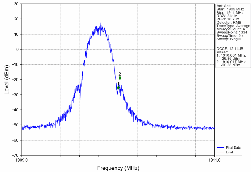
PCS1900_EGPRS_HCH_1909.8MHz_1_TX_Slot_NTNV
