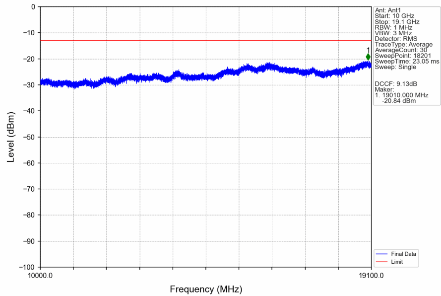
PCS1900_EGPRS_HCH_1909.8MHz_1_TX_Slot_NTNV
