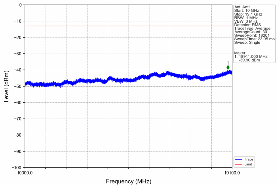
Band2_HSUPA_MCH_1880MHz_Subtest 1_NTNV
