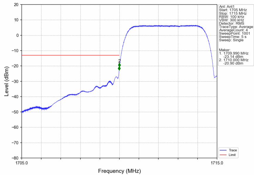
Band4_HSUPA_LCH_1712.4MHz_Subtest 1_NTNV
