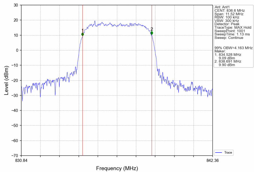
Band5_HSUPA_MCH_836.6MHz_Subtest 1_NTNV
