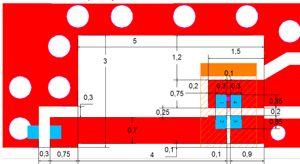
Top Layout(mm)
