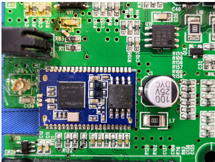
BT&BLE Module
