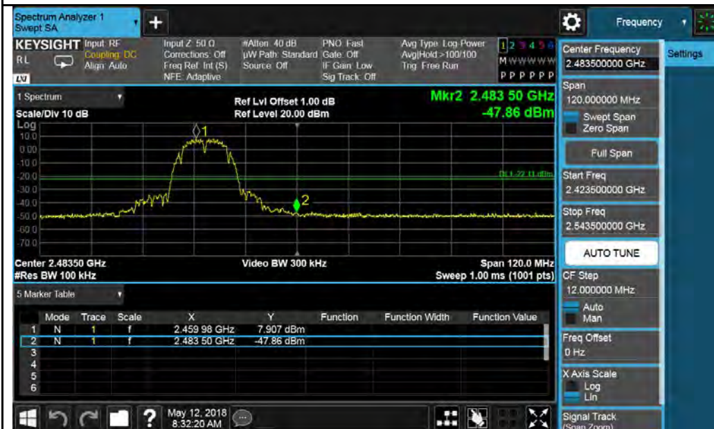
802.11b-2462MHz Chain 1
