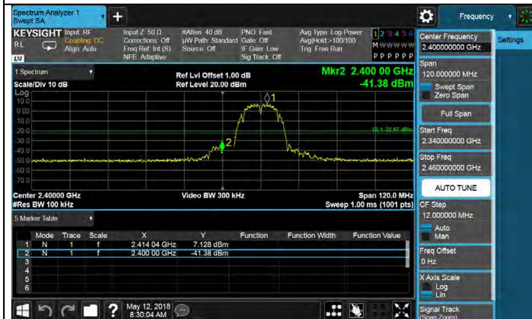
802.11b-2412MHz Chain 1
