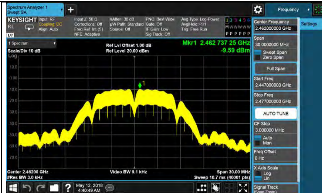
802.11b-2462MHz Chain 0
