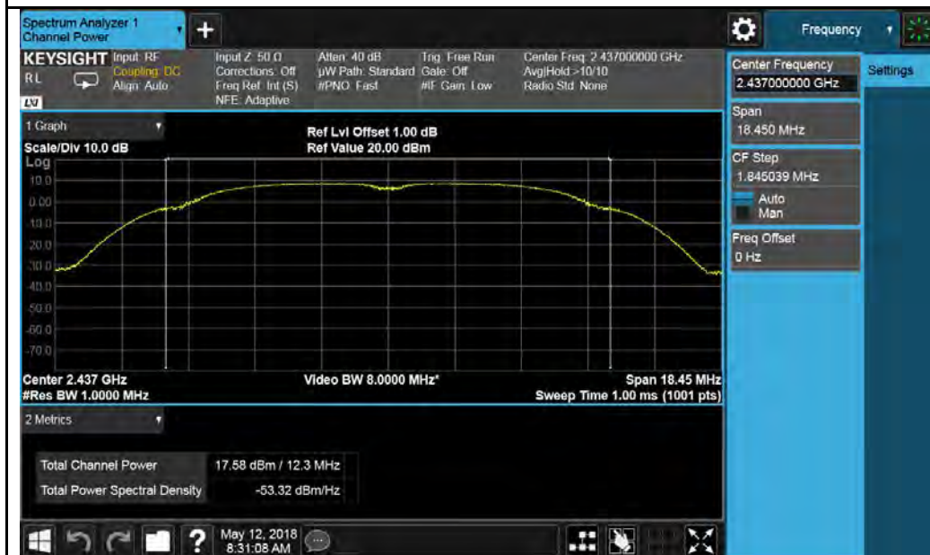
802.11b-2437MHz Chain 1
