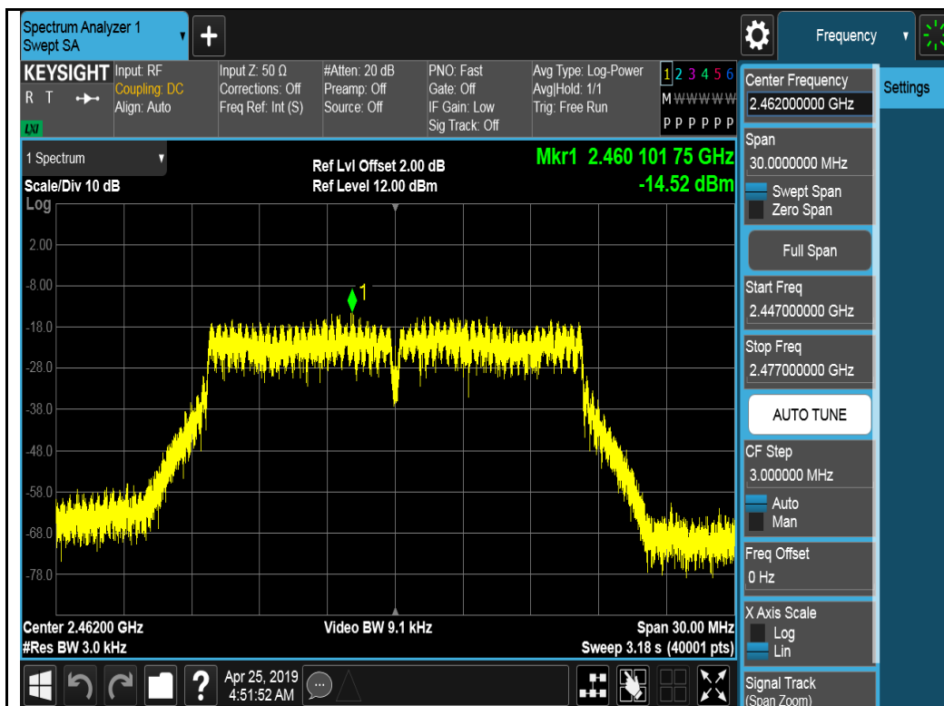
802.11g-2462MHz TX0
