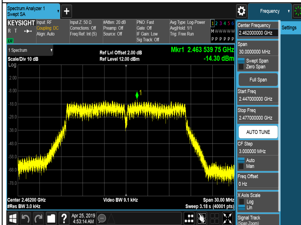
802.11g-2462MHz TX1
