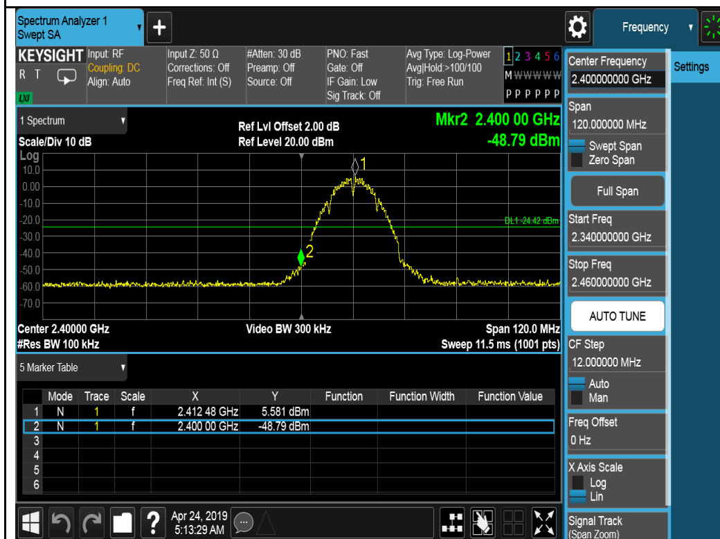
802.11b-2412MHz TX1
