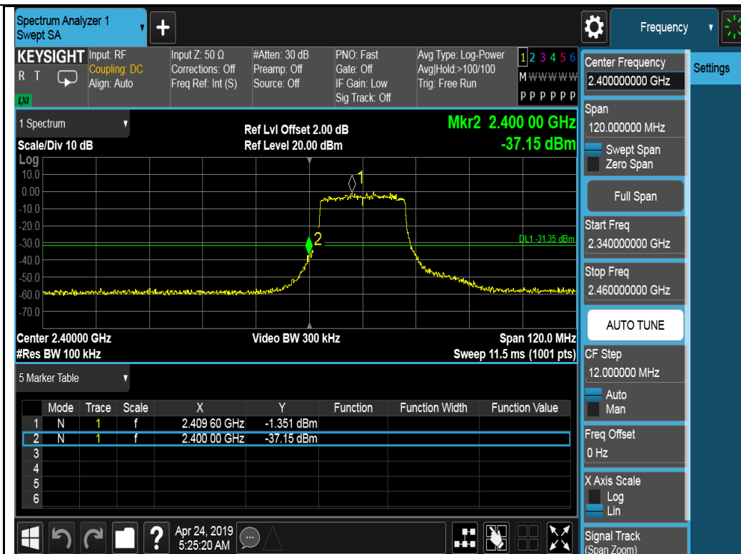
802.11n-HT20-2412MHz TX0
