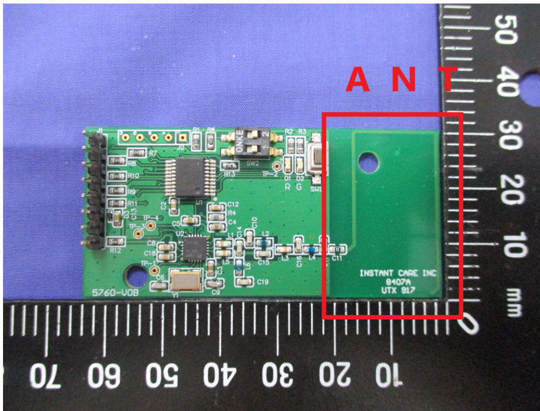
Antenna
