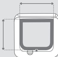
Abmessungen der Klappenöffnung 142 x 120mm (5 5/8" x 4 3/4")
