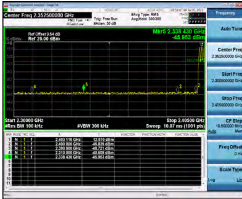
DH5_Low_2402
