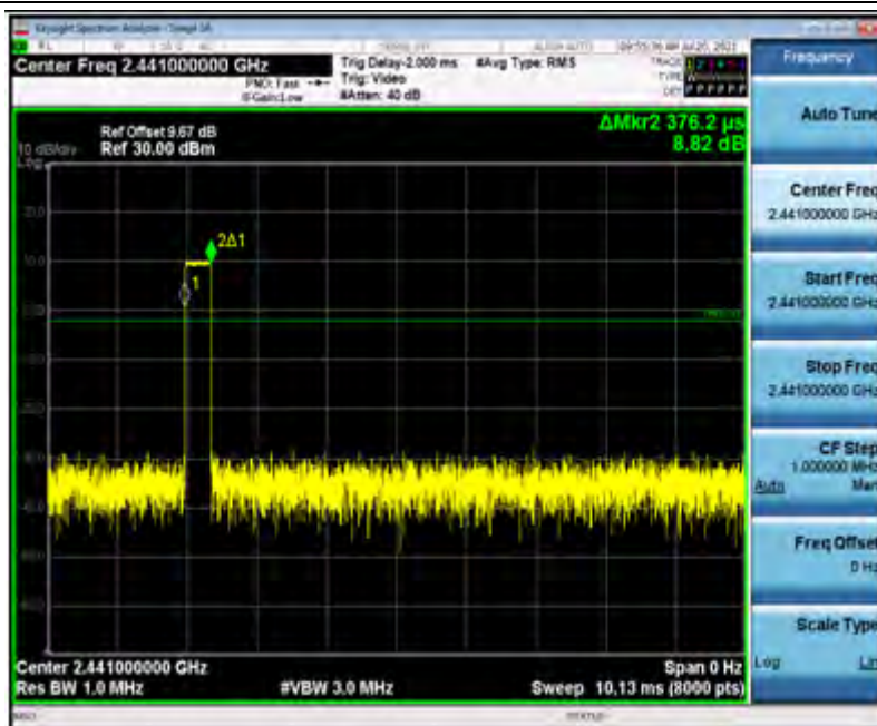
DH1_Hop
