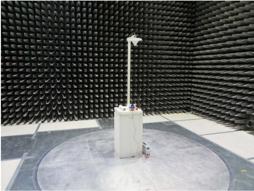
Vee Antenna
