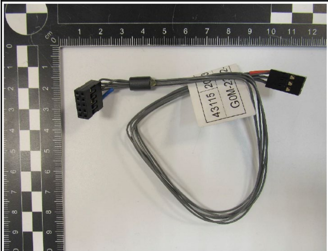
SPI Cable
