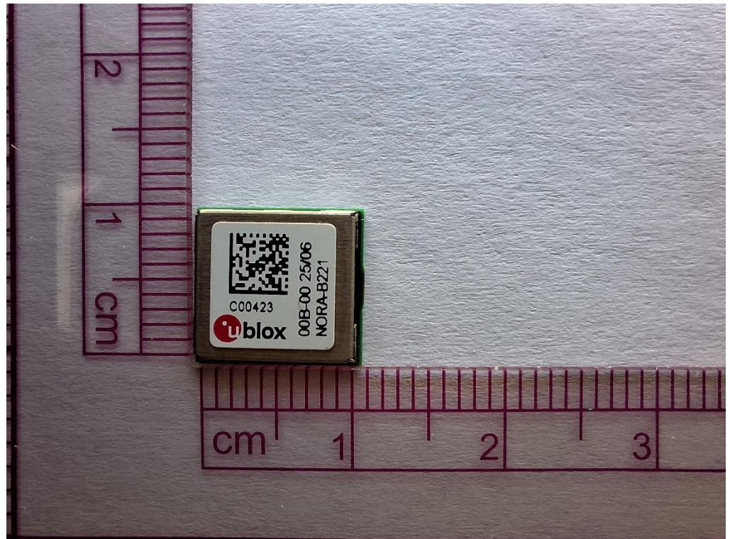
NORA-B221 & NORA-B271
