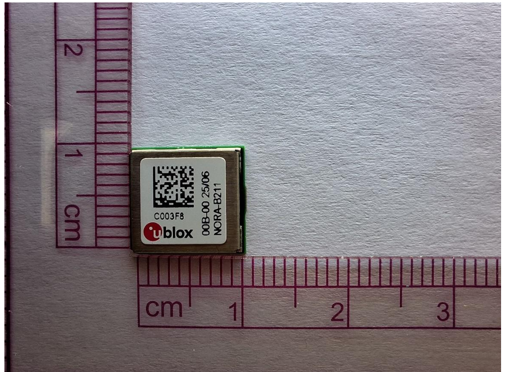
NORA-B211 & NORA-B261
