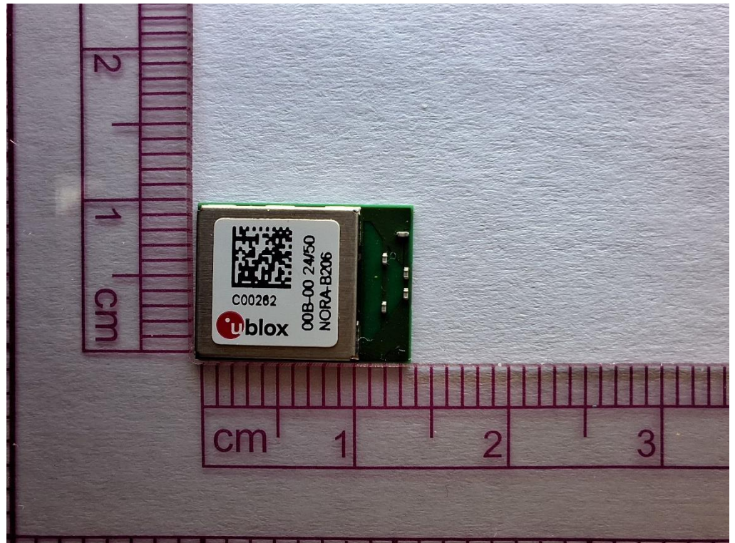
NORA-B206 & NORA-B286
