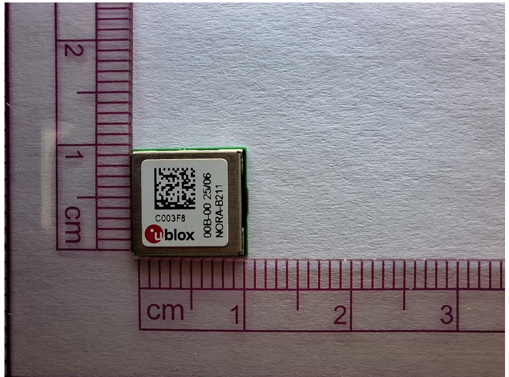
NORA-B211 & NORA-B261
