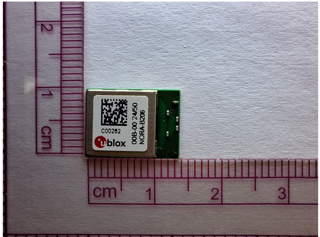
NORA-B206 & NORA-B286
