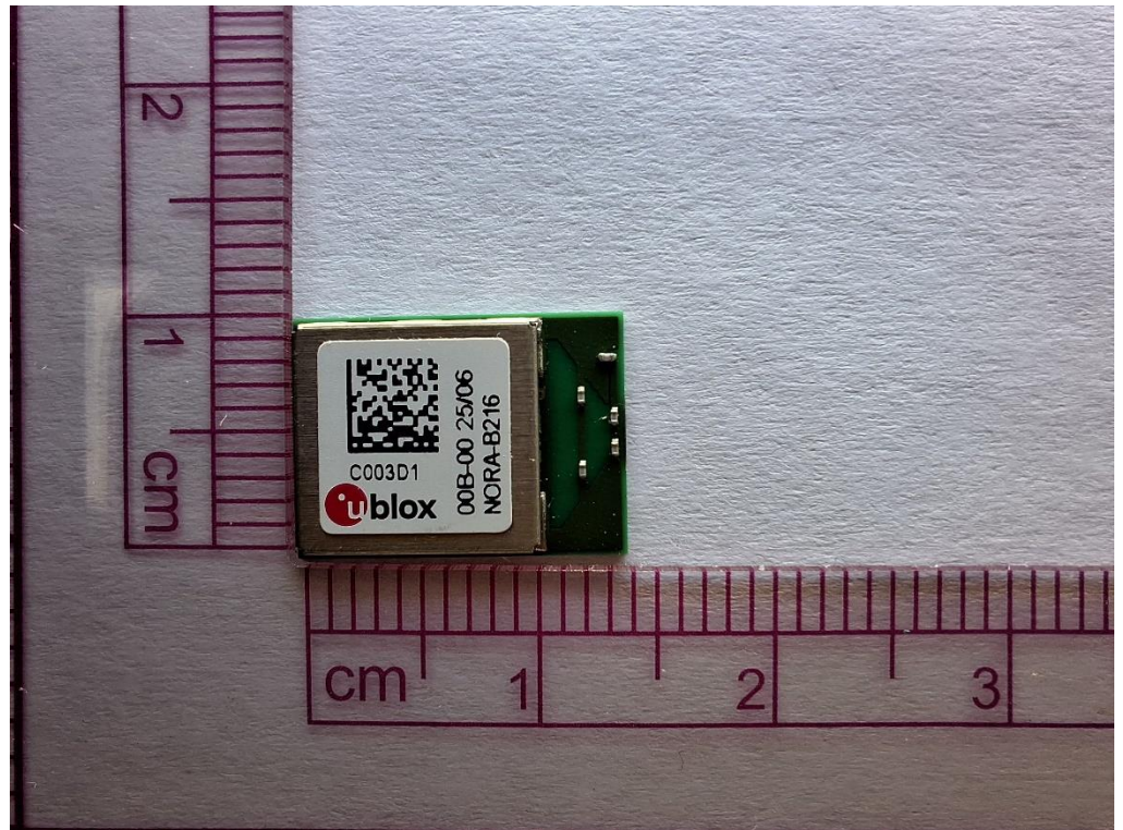
NORA-B216 & NORA-B266
