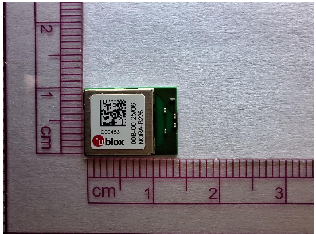
NORA-B226 & NORA-B276
