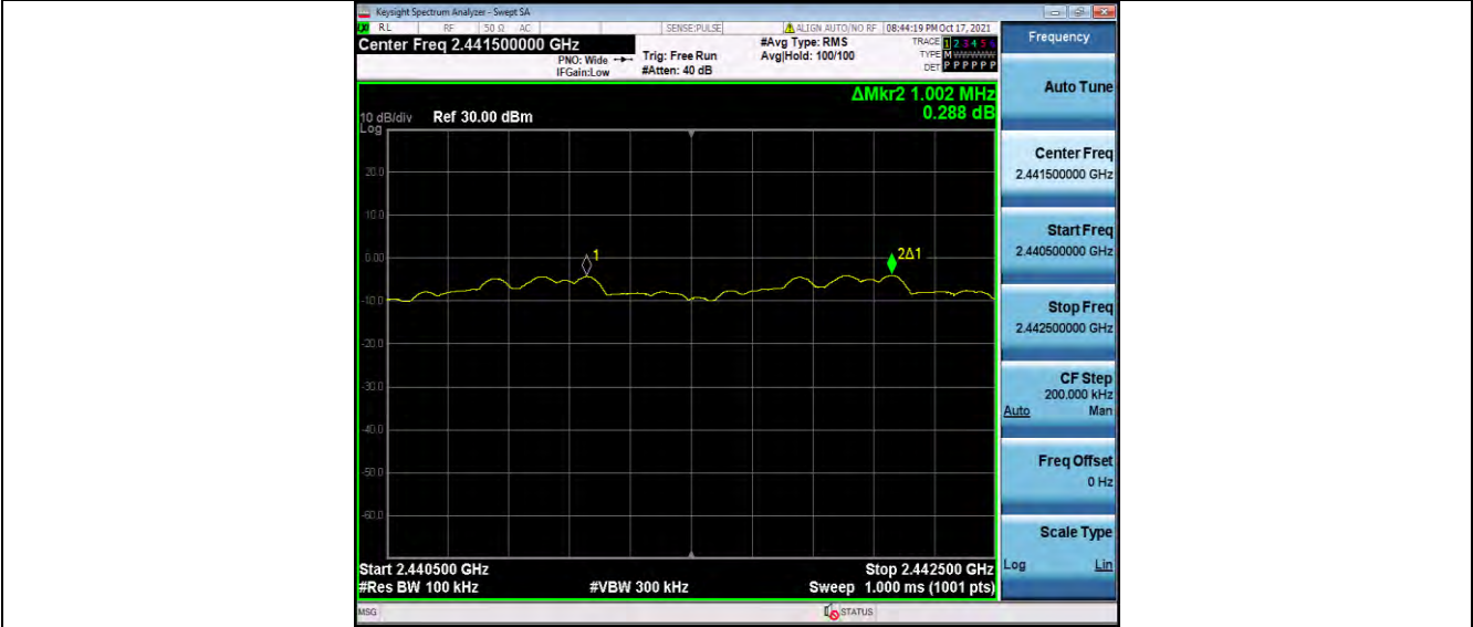
8DPSK
