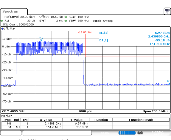
DH1_Hopping_Upper
