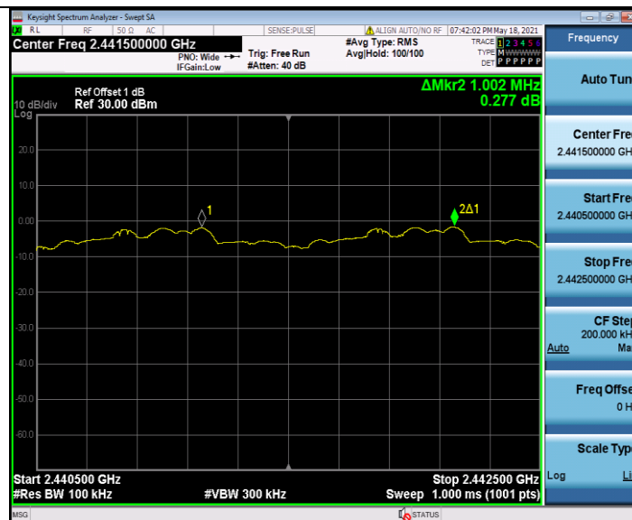
8DPSK
