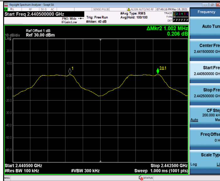
GFSK
