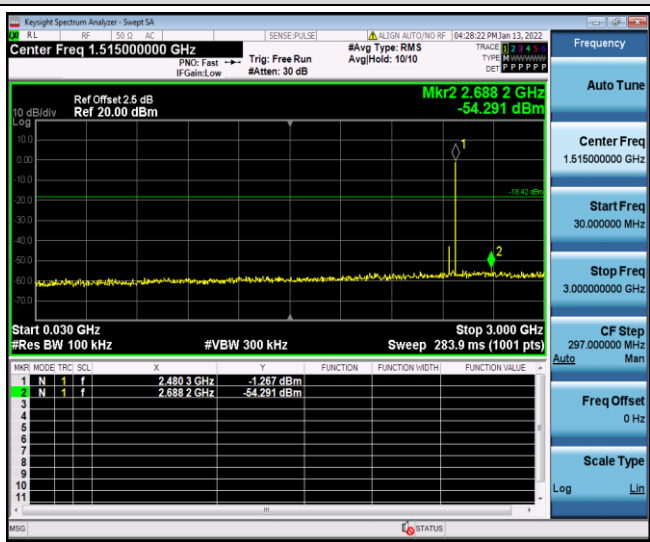
30MHz-3GHz
