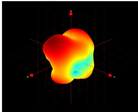
2400MHZ
