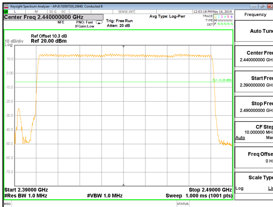
100MHz SPAN
