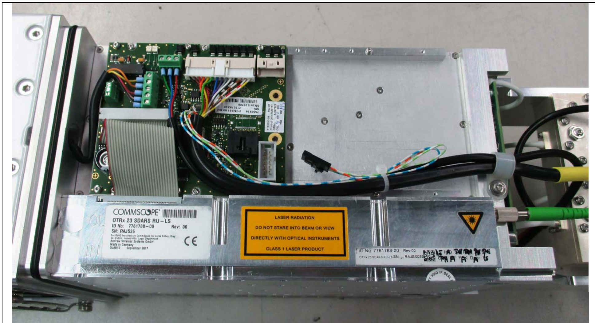
OTRx & Control Board RCM161
