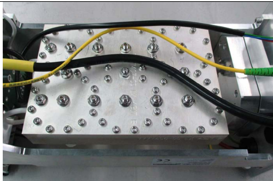
Duplexer
