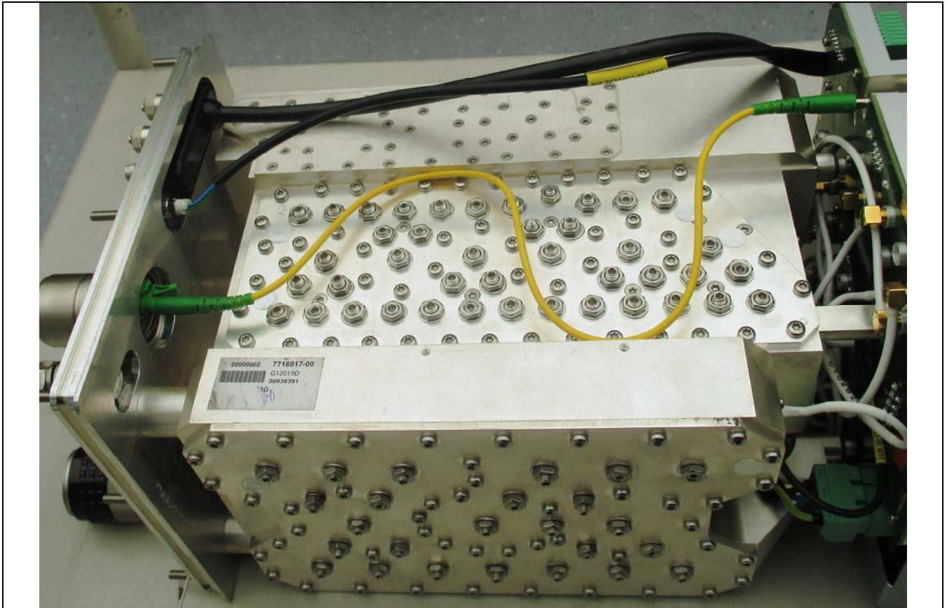
Duplexer
