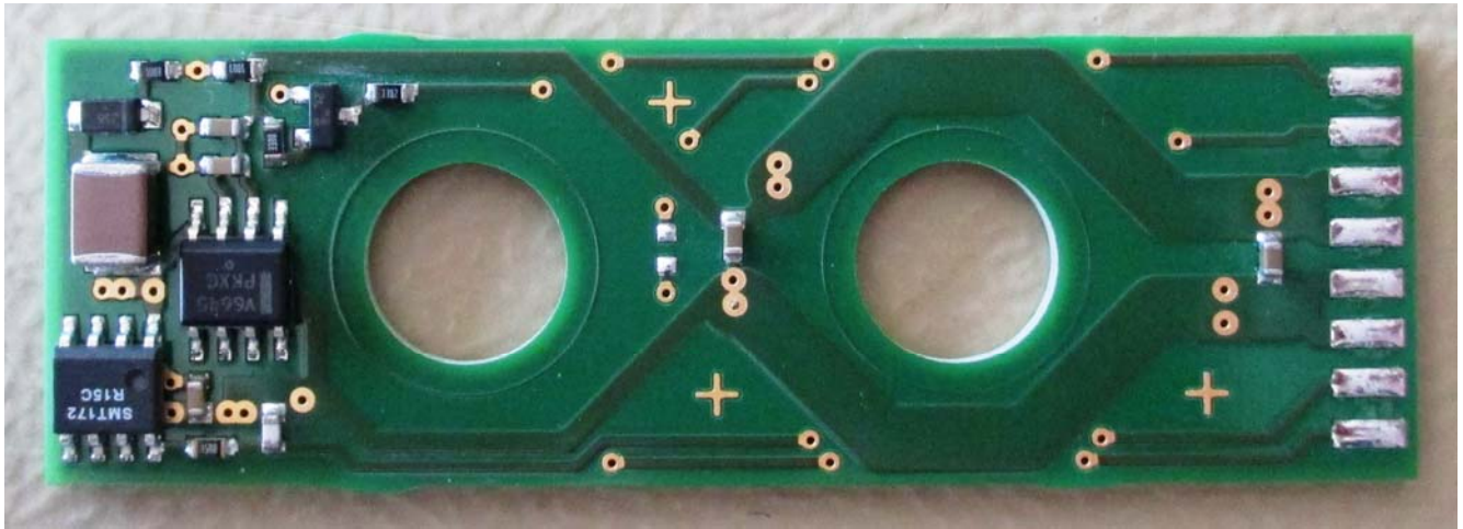
PCB P3683 FanUnitBoard M2-Cab 7659273-01
