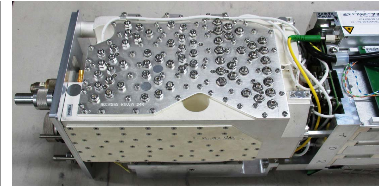
Duplexer
