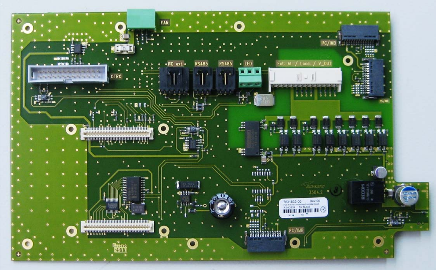
PCB P3504
