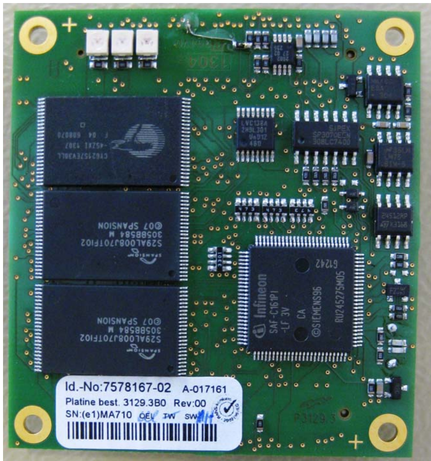
PCB P3129
