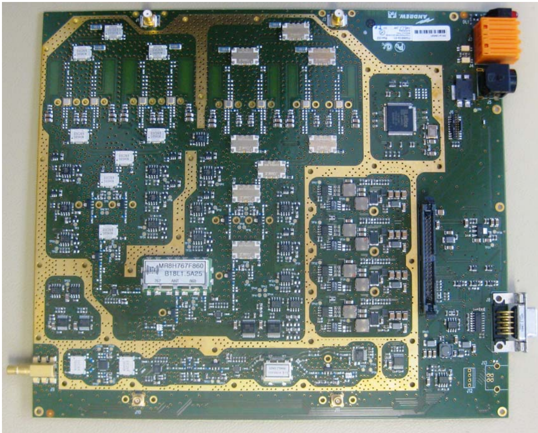
Part 70/80 PCB
