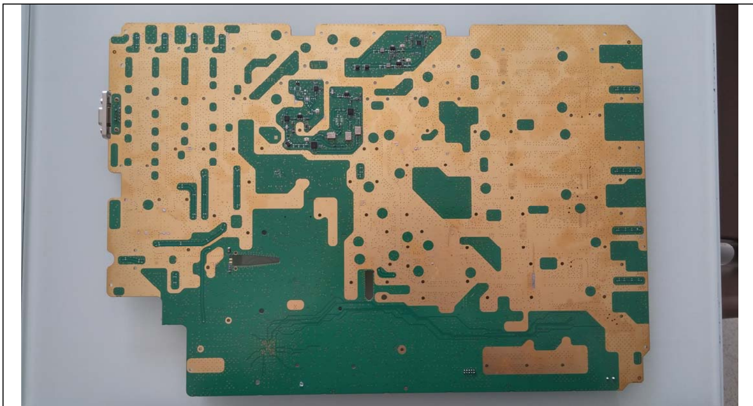
PCB Pop board P3680 ION-U RU US (7714817-00)
