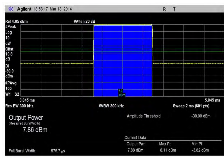
7.2_Max power_UL_1865MHz_GSM
