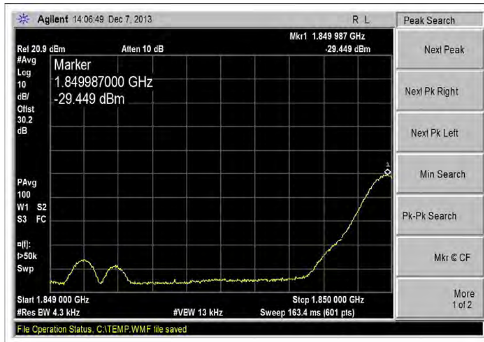
1850 - 1910MHz _ L _ UL GSM, +27dBm
