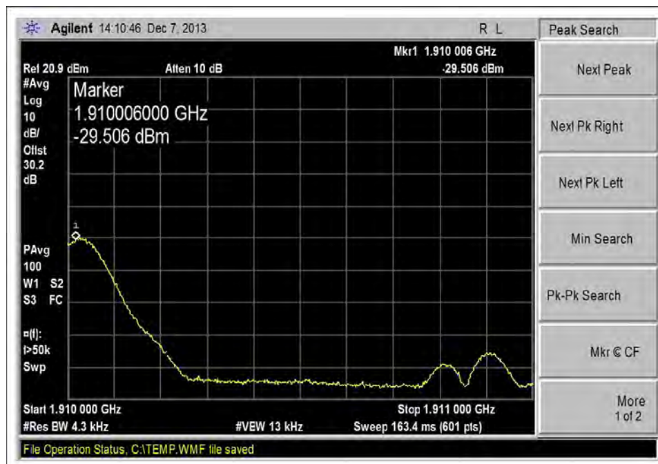
1850 - 1910MHz _ H _ UL GSM, +27dBm
