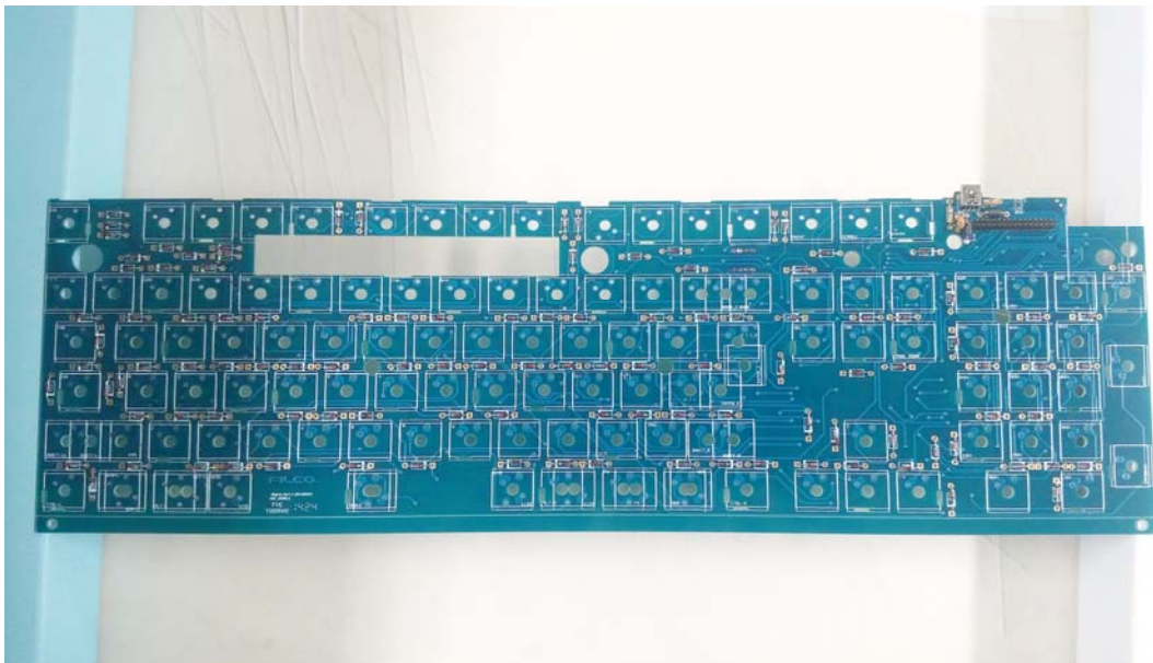
EUT Photo 8 )
